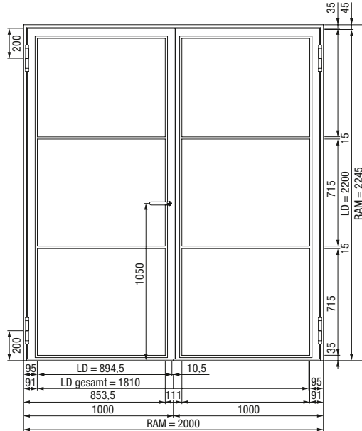
2-flügelige Stahl-Lofttür
